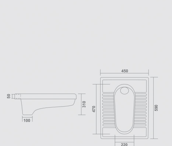
ORISSA PAN - 23" L 450 W 590 H 310mm
